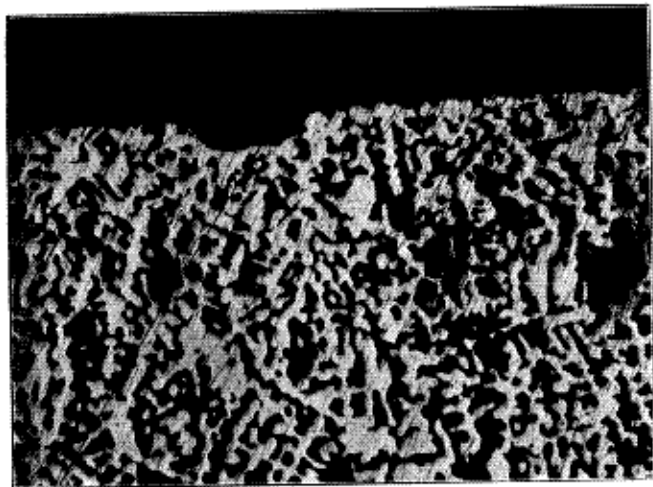
FIG. 4. PORØS BLYPLADE
