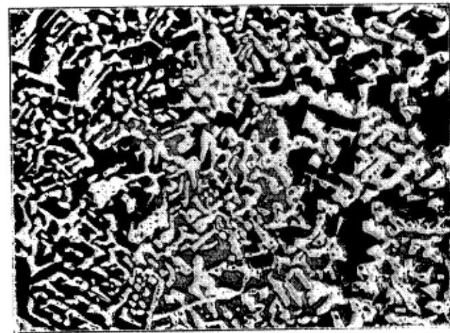
FIG. 6. PORØS ANTIMONPLADE
